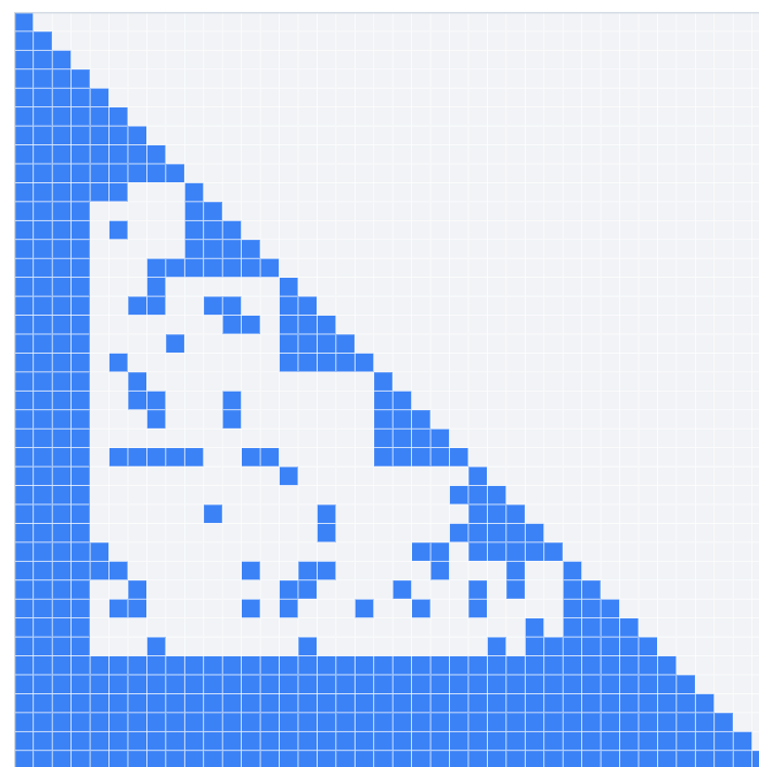
Random-sparse
